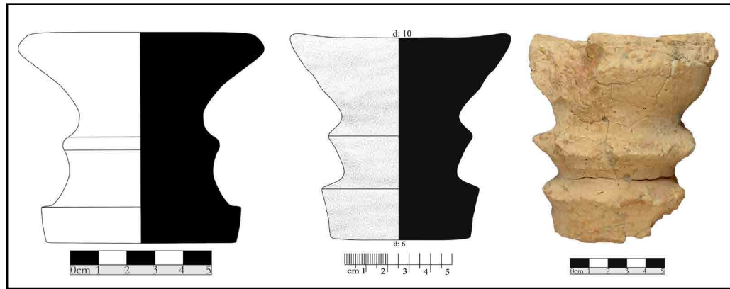
تصویر ۳: گونه ۲ از تپه خواجه خضر (سمت راست) (نگارندگان، ۱۴۰۰) و تل پرگو (سمت چپ) (قنبری و همکاران، ۱۳۹۵: ۲۹۴). Fig. 3: Type 2 of Khajeh Khezr mound (right) (Authors, 2022) and Tol-e Pargo (left) (Ghanbari, Zifar and Gargari, 2016: 294).
