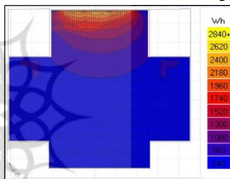
۸. دریافت متوسط تابش روزانه تابستان در فرم چلیپا (کنونی). تابستان نشین خانه لاری‌ها (منبع: نرم افزار اکوتکت). ۳
