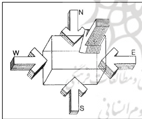
ت ۷. تابش خورشید بر جداره‌های بنا در عرض جغرافیایی ۳۶ درجه (منبع: Mazria, ۱۹۷۹، ۸۱).
