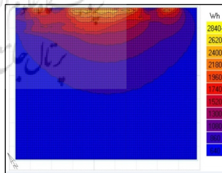
۹. دریافت متوسط تابش روزانه تابستان در فرم مستطیل، با شرایط تابستان نشین خانه لاری‌ها (منبع: نرم افزار اکوتکت).
