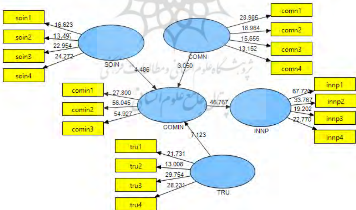
شکل ۴-۲: مدل گرافیکی معناداری ضرایب استاندارد مسیر (تی - والیو)
