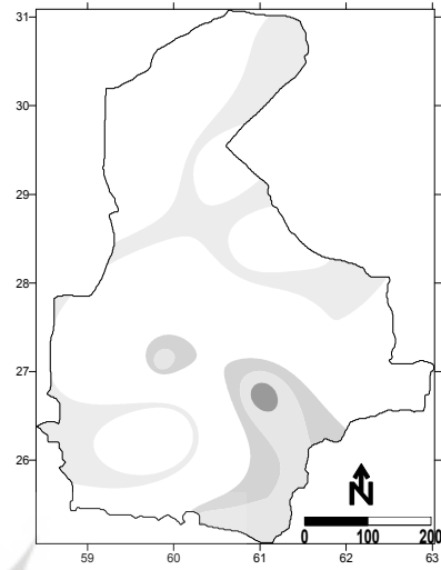
شکل ۷: تحلیل مکانی عامل حرارتی (عامل سوم) شکل ۸: تحلیل مکانی عامل تابشی (عامل چهارم)
