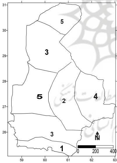
شکل ۹: تحلیل مکانی عامل بادی و تندری (عامل پنجم) شکل ۱۰: نواحی اقلیمی استان سیستان و بلوچستان
