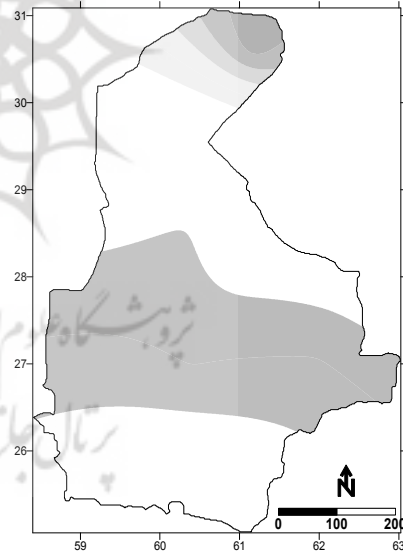
شکل ۹: تحلیل مکانی عامل بادی و تندری (عامل پنجم) شکل ۱۰: نواحی اقلیمی استان سیستان و بلوچستان
