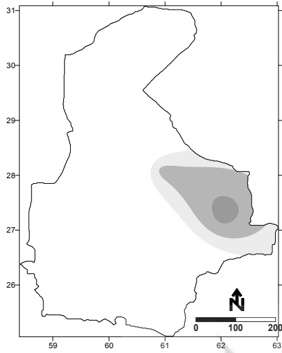
شکل ۷: تحلیل مکانی عامل حرارتی (عامل سوم) شکل ۸: تحلیل مکانی عامل تابشی (عامل چهارم)
