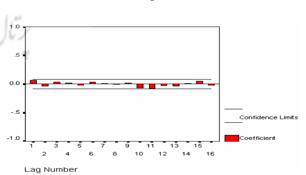
شکل ۸- نمودار تابع خود همبستگی باقیمانده های بارش ماهانه بیرجند
