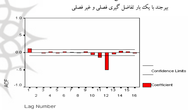
شکل ۶- نمودار تابع خود همبستگی سری زمانی بارش ماهانه بیرجند با یک بار تفاضل گیری فصلی و غیر فصلی
