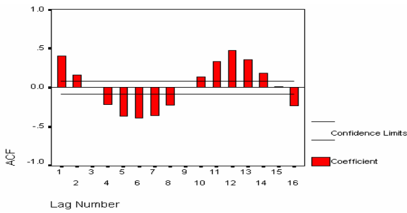
شکل ۳- نمودار تابع خود همبستگی سری زمانی بارش بیرجند
