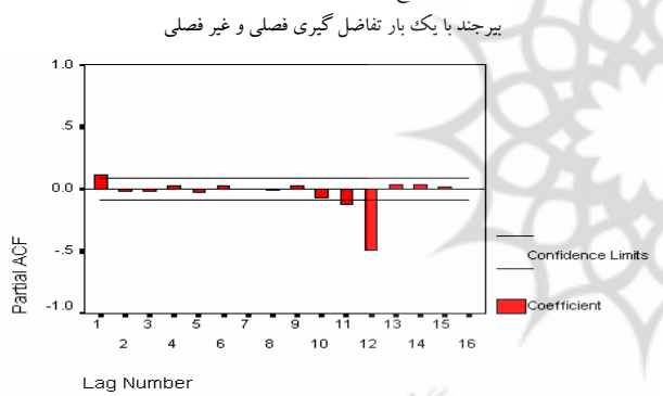
شکل ۷- نمودار تابع خود همبستگی جزئی سری زمانی بارش ماهانه بیرجند با یک بار تفاضل گیری فصلی و غیر فصلی
