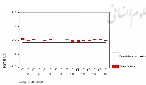
شکل ۹- نمودار تابع خود همبستگی جزئی باقیمانده های بارش ماهانه بیرجند
