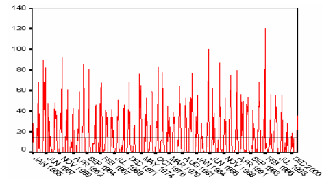
شکل ۲- نمودار سری های زمانی داده های اصلی بارش ماهانه بیرجند
