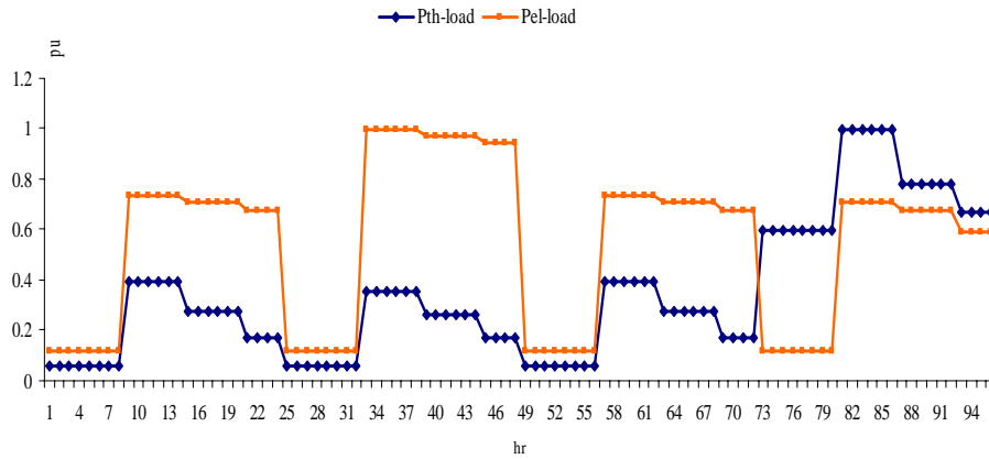
شکل ۵ - منحنی بار الکتریکی و حرارتی ۲۴ ساعته یک روز از هر فصل (۲۴-۰، بهار، ۴۸-۲۵، تابستان، ۷۲-۴۹، پاییز و ۹۶-۷۳، زمستان) برای بیمارستان به صورت پرونیوت
