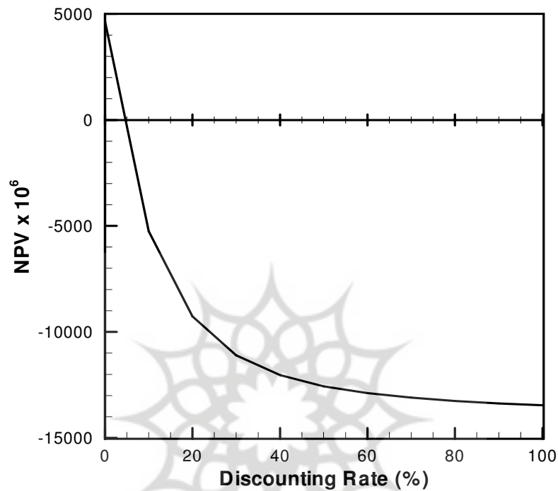
شکل ۲. ارزش فعلی خالص با توجه به نرخ تنزیل‌های مختلف برای سرمایه‌گذار با استفاده از نرم‌افزار COMFAR EXPERT III
