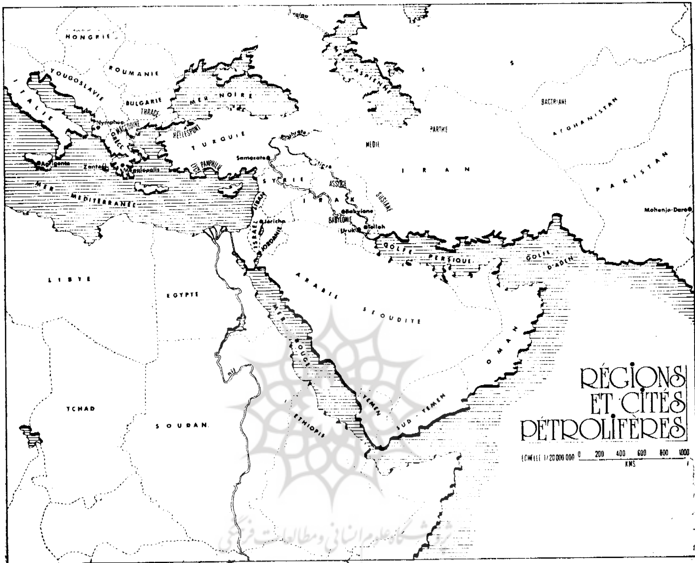
نواحی و شهرهای نفتخیز دوران باستان
