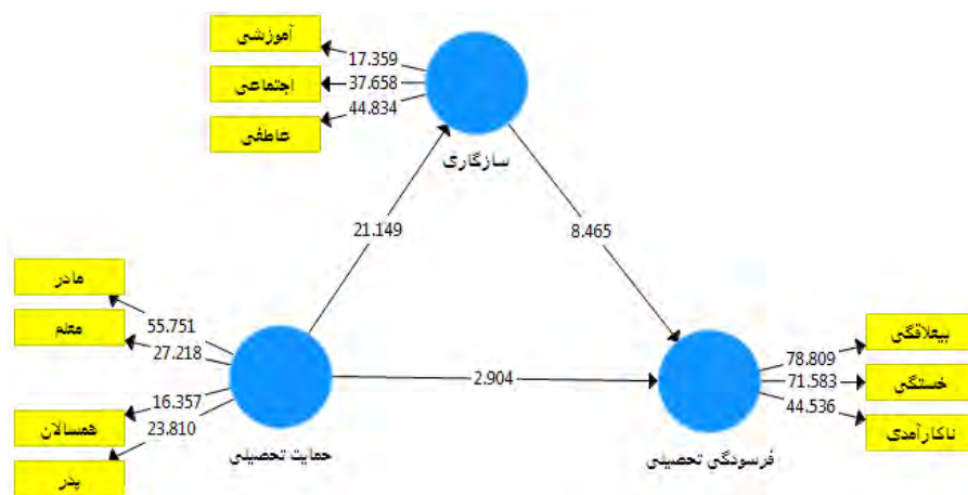
شکل ۲) مدل آزمون شده متغیرهای پژوهش بر مبنای T-value
