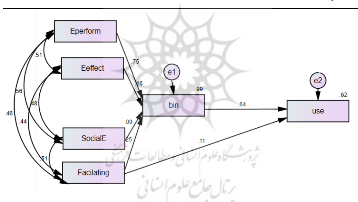
نمودار ۱. نمودار مسیر پیش بینی براساس ضرایب مسیر استاندارد شده
