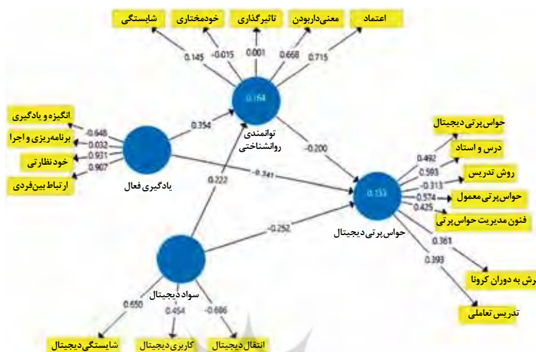
شکل ۲. ضرایب مسیر
