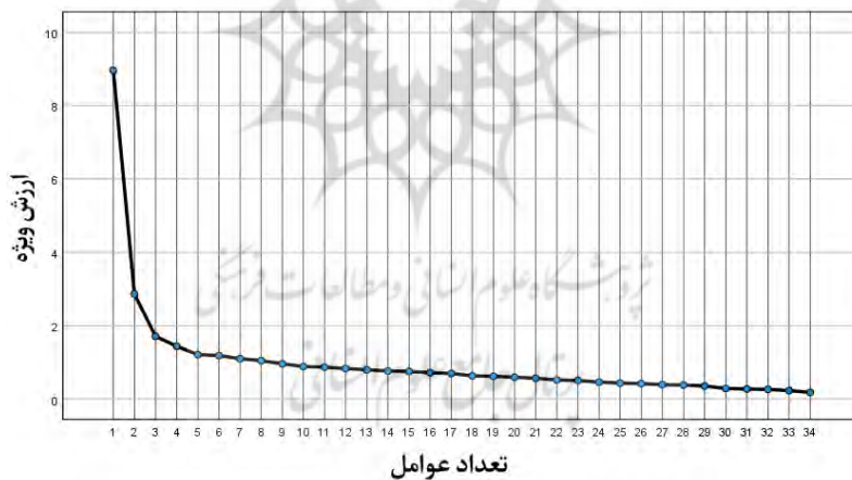
شکل ۱: نمودار سنگ‌ریزه برای تعیین تعداد عوامل در مقیاس فرهنگ مهدویت
