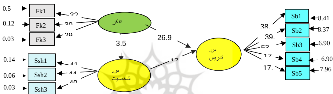
شکل ۵: مدل ساختاری کلی
