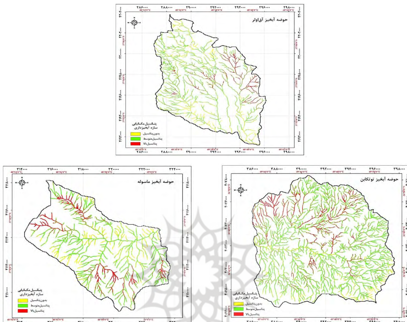
شکل (۸): نقشه نهایی مکان‌یابی احداث سازه‌های آبخیزداری (گابیون و سنگی‌ملاتی) در حوضه‌های آق‌اولر، توتکابن و ماسوله
