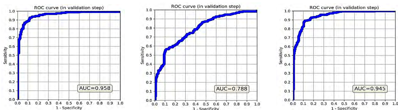
شکل (۹): منحنی تشخیص عملکرد (ROC) و سطح زیر منحنی (AUC) حوضه‌های آبخیز آق‌اولر (راست)، توتکابن (وسط) و ماسوله (چپ)
