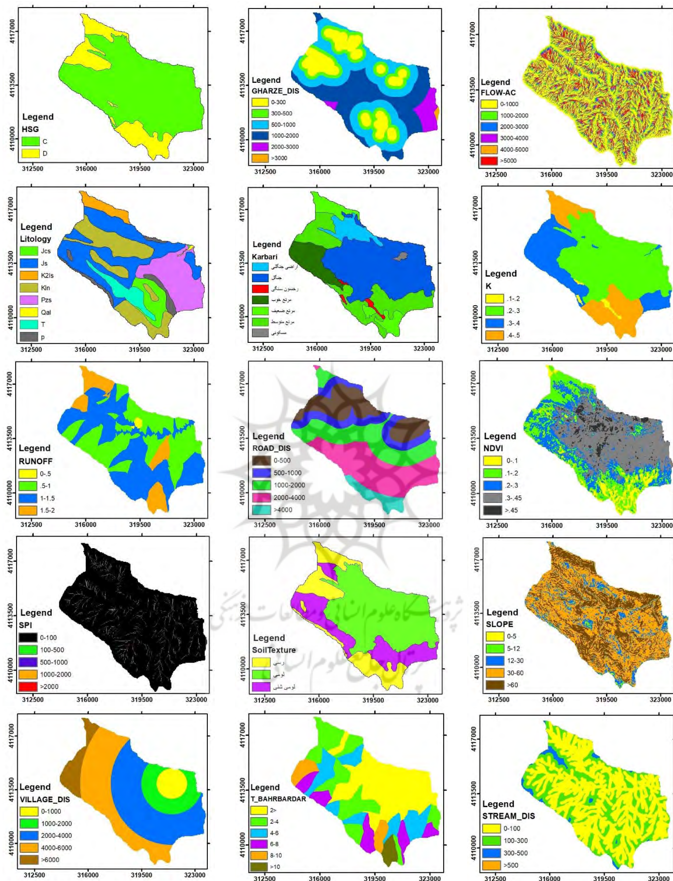
ادامه شکل (۵): نقشه معیارهای تأثیرگذار روی مکان‌یابی سازه‌های آبخیزداری در حوضه آبریز ماسوله
