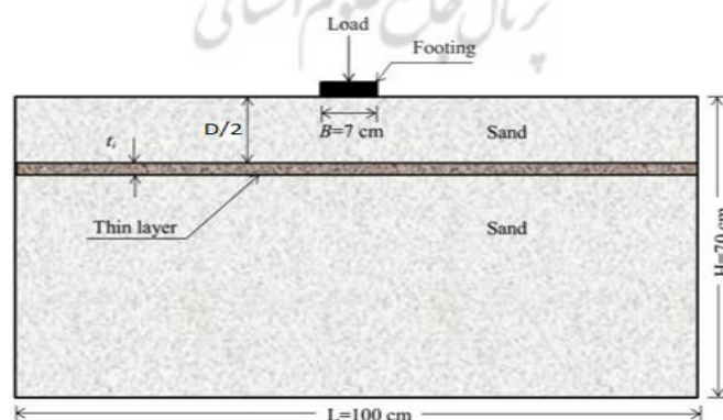
شکل ۲. هندسه مدل جهت آنالیز المان محدود.
