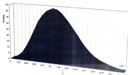
شکل ۴. هیدروگراف واحد مصنوعی خروجی زیر حوضه نخل ناخدا
