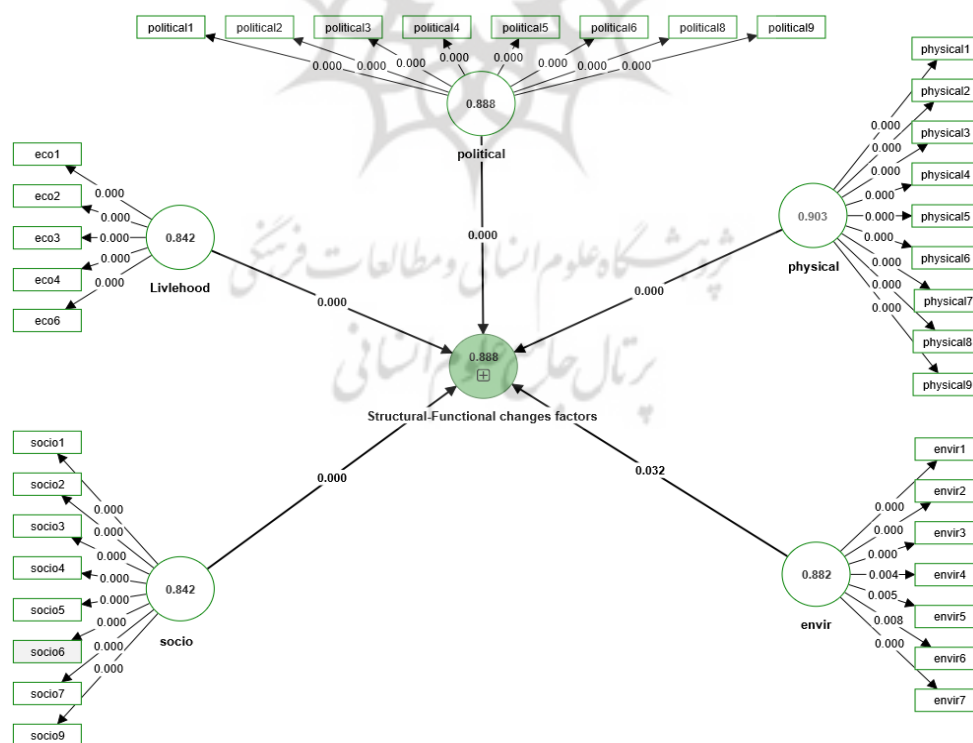
شکل ۴. مدل مؤلفه‌های سلسله‌مراتبی با مقدار P-Value
