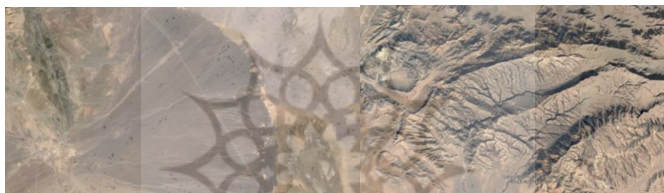
شکل ۵. مخروط افکنه
