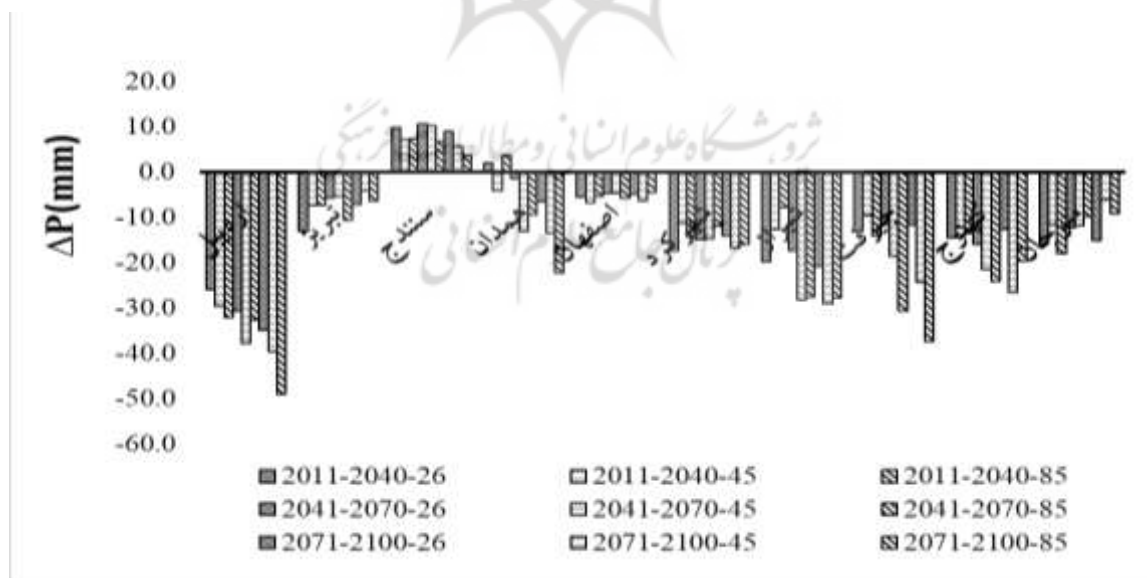
شکل ۶. تغییرات بارش سالانه در سه دوره ۲۰۱۱-۲۰۴۰، ۲۰۴۱-۲۰۷۰ و ۲۰۷۱-۲۰۱۰۰ تحت سه سناریوی انتشار RCP2.6، RCP4.5 و RCP8.5
