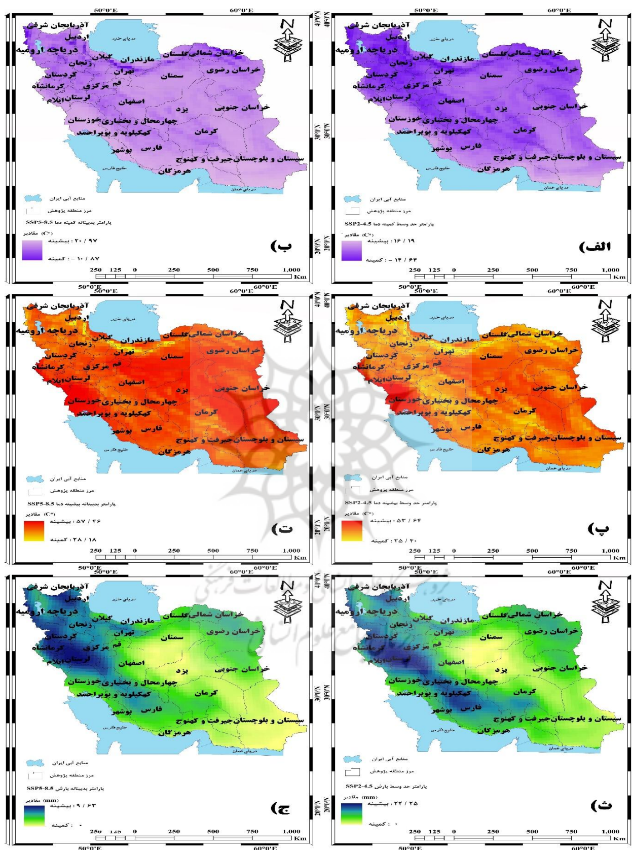
شکل ۵. نقشه‌های تصاویر ماهواره‌ای پیش‌بینی عناصر اقلیمی کمینه دما، بیشینه دما و بارش بر پایه سناریوهای حد وسط SSP2_4.5 و خیلی بدبینانه SSP5_8.5، در دوره آینده دور (۲۰۶۱-۲۱۰۰) براساس مدل CanESM5
