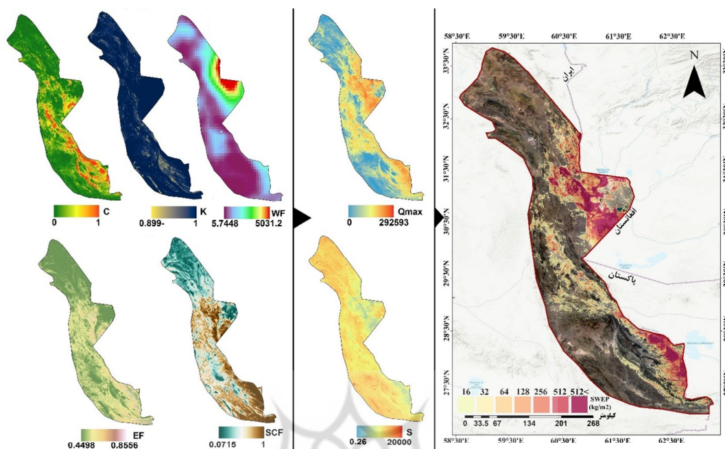
شکل ۳. پتانسیل فرسایش بادی (SWE)، همراه با عامل‌های C (ضریب پوشش گیاهی)، K (ضریب زبری خاک)، WF (عامل اقلیم)، EF (جزء فرسایش‌پذیر) و SCF (ضریب پوسته خاک)
