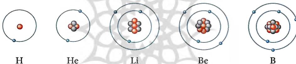
شکل ۲- مدل اتمی بور برای اتم‌های هیدروژن، هلیوم، لیتیم، بریلیم و بور
