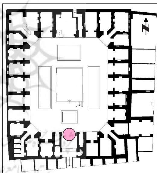
● موقعیت فضای نیایش (نمازخانه) در پلان مدرسه التفاتیه نمازخانه مدرسه التفاتیه از وسعت کمی برخوردار بوده و کارکرد عمومی ندارد. سمت چپ بالا: تصویر نمازخانه مدرسه (عکس: نگارنده، ۱۳۹۰)
