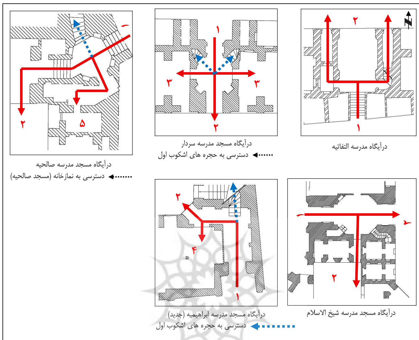
شکل ۱۸. ارتباط درآیگاه با میانسرا، فضای زندگی، فضای آموزش و فضای نیایش در مدرسه‌های قزوین. ۱- درآیگاه ۲- میانسرا ۳- مدرس ۴- نمازخانه ۵- حجره (منبع پلان‌ها: مرکز اسناد اداره کل میراث فرهنگی استان قزوین، ۱۳۸۹، سند شماره ۱۰۵-۱۰۱)
