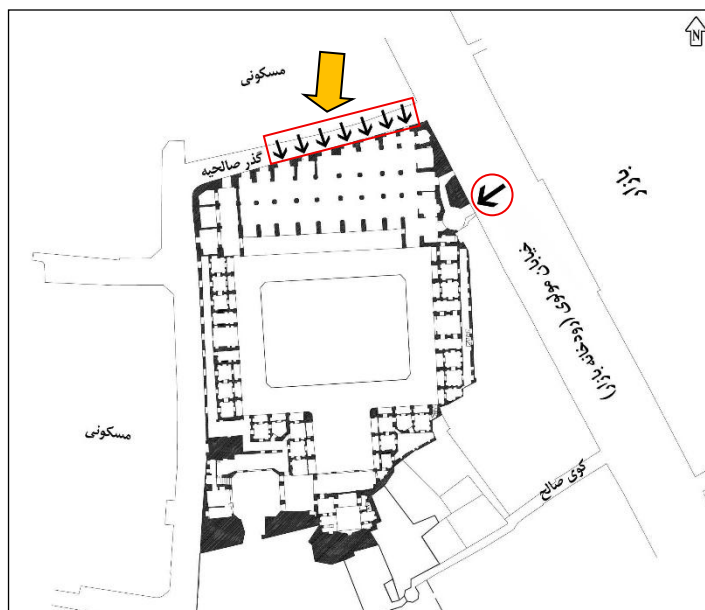
شکل ۹. پلان معماری اشکوب همکف مسجد مدرسه صالحیه قزوین (منبع: مرکز اسناد اداره کل میراث فرهنگی استان قزوین، ۱۳۸۹، سند شماره ۱۰۳) ایجاد بیش از هفت دسترسی مستقیم (بدون فضای واسطه) به فضای نیایش (یا همان مسجد صالحیه) از گذر شمالی صالحیه جهت ورود و خروج عموم مردم به منظور عدم تداخل با فضای زندگی و درس طلاب
