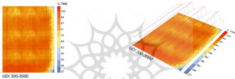
شکل ۹. نحوه توزیع یکنواخت نور روز سالن ورزشی پس از انجام بهینه‌سازی و دریافت میانگین % ۸۳.۵۷ نور بهینه (مأخذ: نگارندگان)
