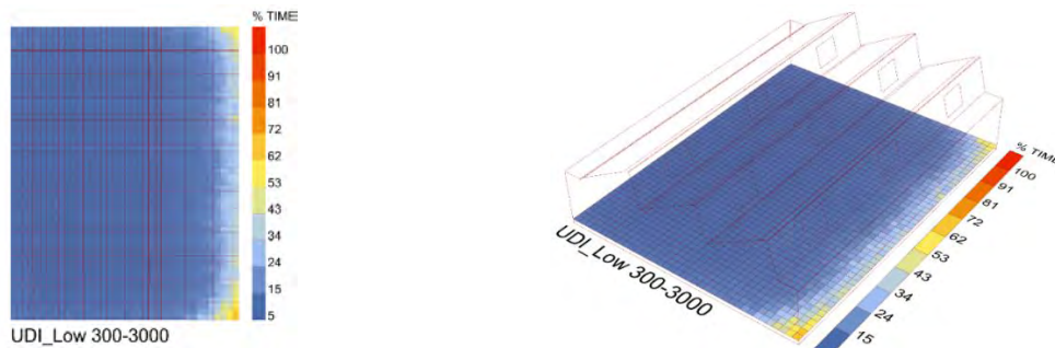
شکل ۱۱. خروجی نرم‌افزار روشنایی مفید نور روز، میانگین کمبود دریافت نور مناسب در سالن ورزشی % ۹.۸۵ است (مأخذ: نگارندگان)
