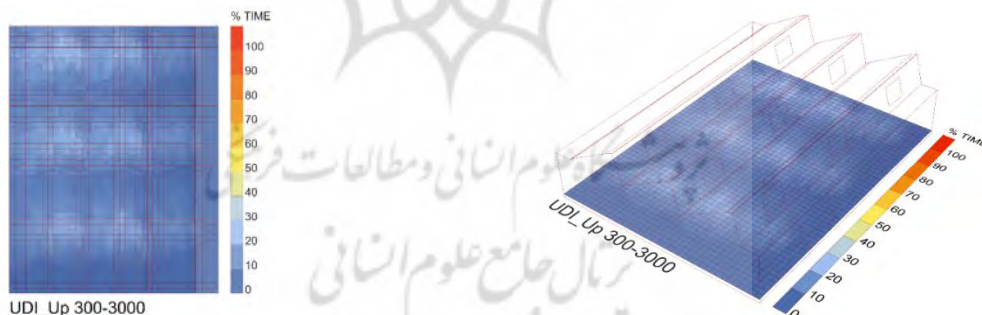
شکل ۱۰. خروجی نرم‌افزار روشنایی مفید نور روز، میانگین خطر احتمال بروز خیرگی در سالن ورزشی % ۶.۵۸ است (مأخذ: نگارندگان)
