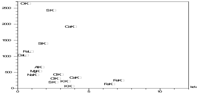
شکل ۳. طیف تجزیه عنصری نمونه A
