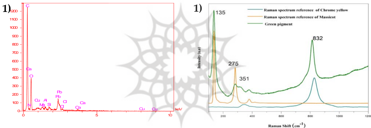
شکل ۴. آنالیز عنصری SEM-EDS حاصل از رنگ‌دانه سبز (۱)، طیف رامان رنگ‌دانه سبز نمونه و طیف مرجع رنگ‌دانه زرد کروم و ماسیکوت (۲).
