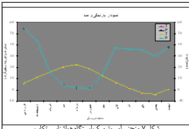
شکل ۷ منحنی امبروترمیک ایستگاه هواشناسی تکاب
