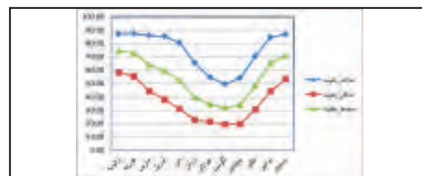
شکل ۹. نمودار میانگین حداکثر، حداقل و متوسط رطوبت نسبی ماهانه دوره آماری (۱۹۹۰-۲۰۲۳) بر حسب درصد Fig 9. Diagram of the average maximum, minimum, and relative humidity for the monthly period of 2023-1990 (in percentage).
