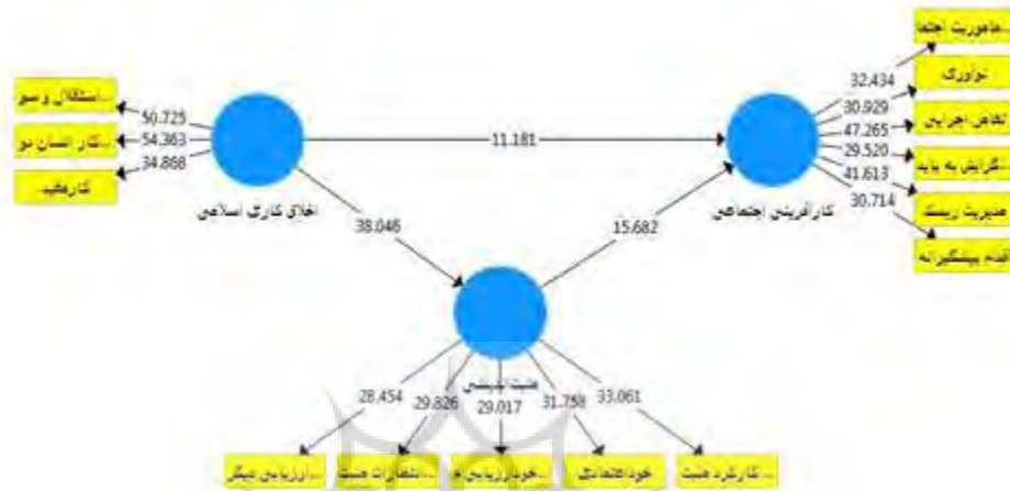
شکل ۳. مقدار آماره t برای بررسی معنی داری ضرایب مسیر و بارهای عاملی مأخذ: یافته‌های پژوهش (۱۴۰۳)
