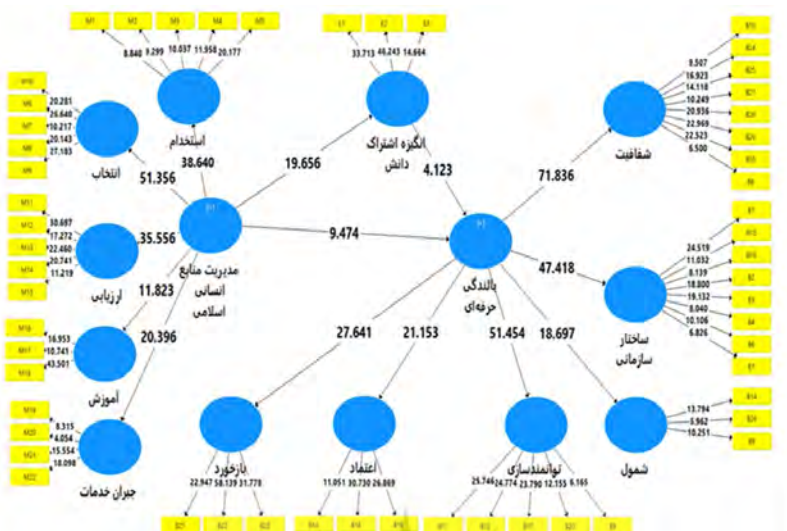
شکل ۳. مدل ساختاری در حالت معناداری ضرایب
