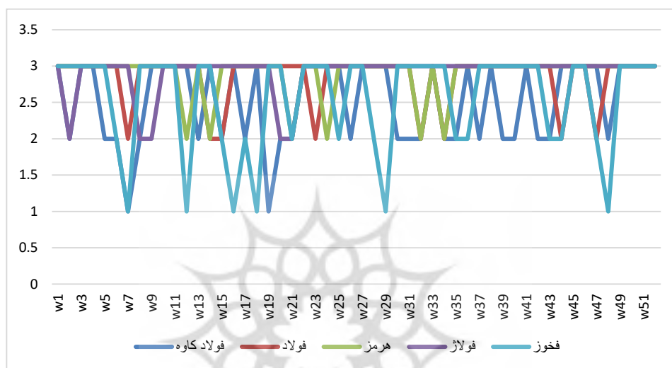
نمودار (۱) - پیش بینی روند قیمت سهام شرکت مورد مطالعه با استفاده از تکنیک ماشین بردار پشتیبان
