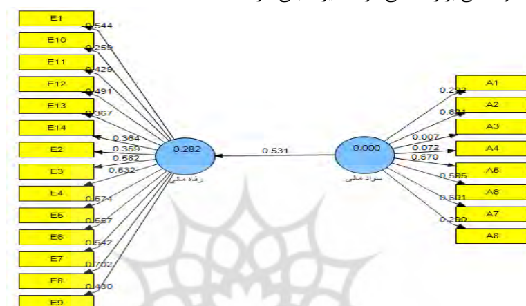
نمودار ۱- تحلیل عاملی تاییدی در حالت استاندارد فرضیه اول
