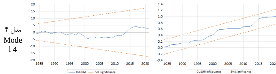
نمودار (۱) نتایج آزمون‌های CUSUM و CUSUMQ Figure (1) Results of CUSUM and CUSUMQ tests
