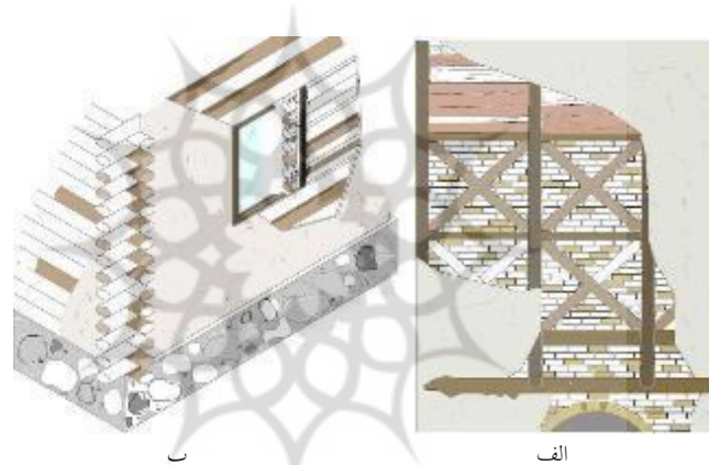
شکل ۱۵: الف: جزئیات یک دیوار قدیمی با سیستم قاب چوبی در ایران ب: جزئیات سیستم دیواردارورچین (نگارندگان، ۱۴۰۳) Fig. 15. A: Details of an old wall with a wooden frame system in Iran B: Details of the Darvarchin wall system (Authors, 2024)
