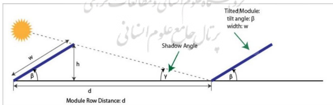
شکل ۳. نمودار تعیین فاصله بهینه بین ردیف‌های پنل‌های خورشیدی بر اساس موقعیت خورشید و تحلیل سایه‌اندازی [۲۳].
