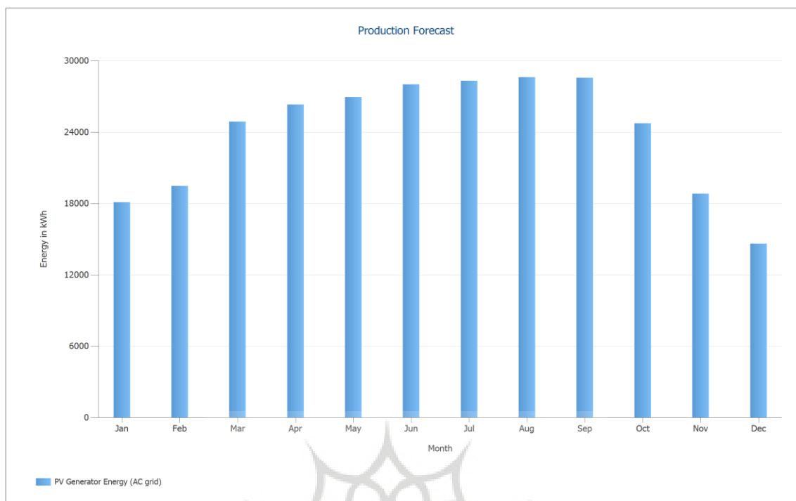
شکل ۸. نمودار پیش‌بینی تولید ماهانه انرژی سامانه فتوولتائیک
