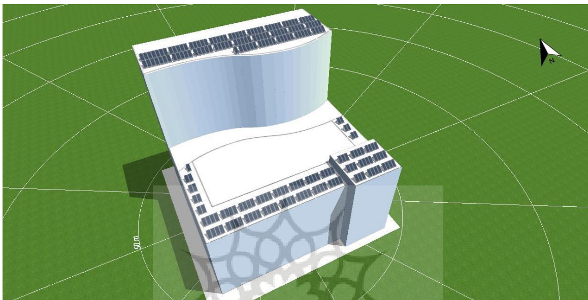
شکل ۵. مدل سه بعدی ساختمان و جانمایی پنل ها بر روی بام
