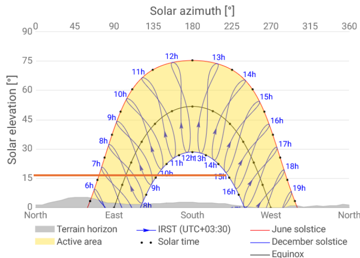
شکل ۴. نمودار مسیر خورشیدی شهر تبریز (Sun path diagram) [۲۴].
