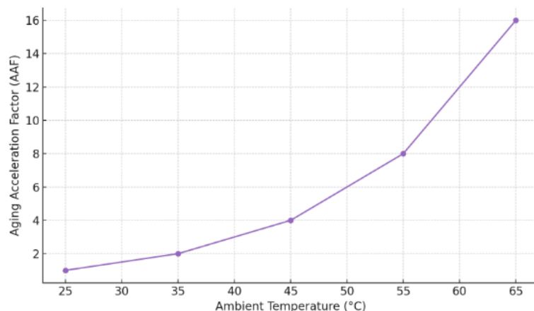
شکل ۸. شتاب گیری نرخ پیری ترانسفورماتور با افزایش دما
