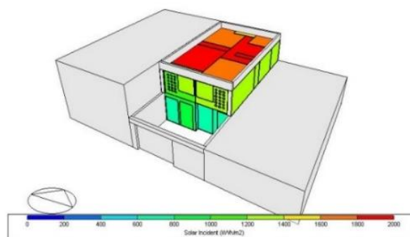
شکل ۶. میزان دریافتی نور خورشید بدون سایبان
