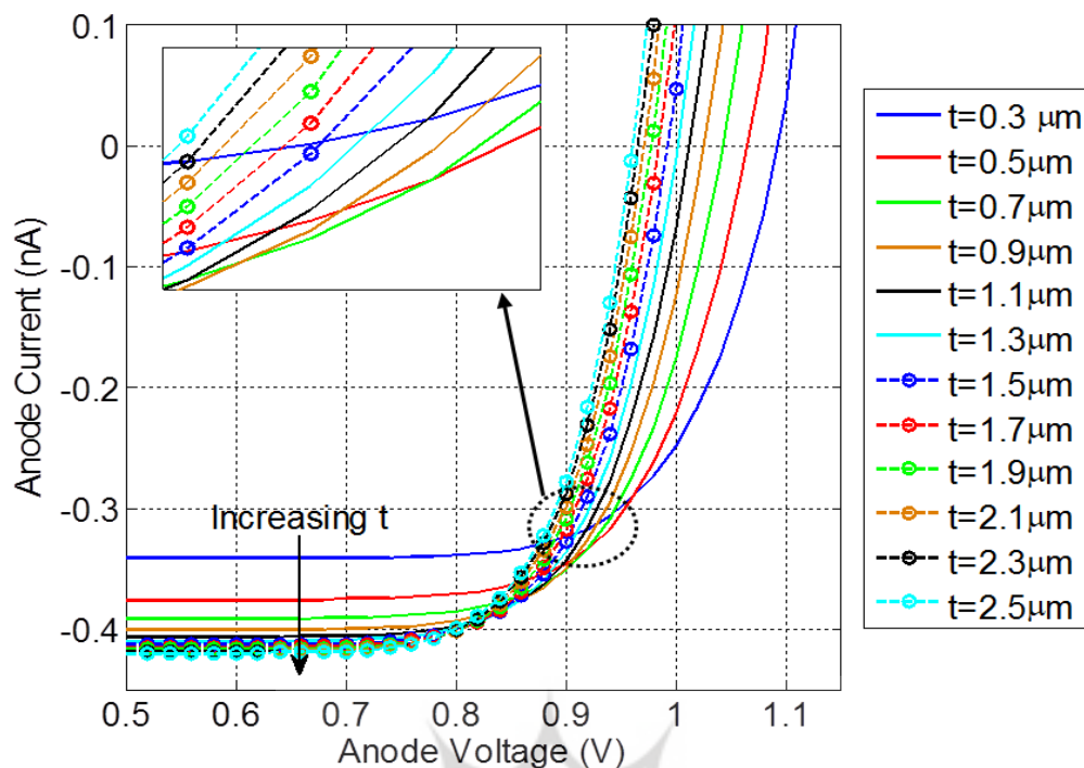
شکل ۳: ضخامت‌های مختلف لایه های جاذب درجه بندی شکاف نواری (قسمت Pmax در نمودار بزرگنمایی شده است) همانطور که در شکل (۴) مشاهده می شود، با افزایش ضخامت لایه های جاذب، V_{oc} در حال کاهش است، به نظر می رسد که این امر به دلیل افزایش نرخ نوترکیبی با افزایش ضخامت باشد که بر جریان اشباع تاریک تاثیر گذاشته و باعث افت ولتاژ مدار باز سلول شده است. همچنین با افزایش ضخامت لایه های جاذب، سرعت تولید در لایه های جاذب افزایش می یابد و منجر به افزایش جریان اشباع اتصال کوتاه سلول می شود (همانطور که در شکل (۴) نشان داده شده است). همه این اتفاقات که در سلول رخ می دهد همراه با دلایل افزایش ضریب پر شدگی سلول منجر به افزایش کارایی سلول گردیده و در 1/3 میکرومتر به مقدار بهینه رسیده است
