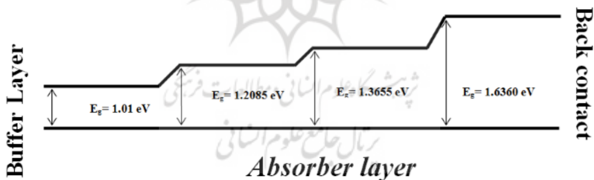
شکل ۲: پروفیل‌های باند شکاف جذاب سلول خورشیدی CIGS
