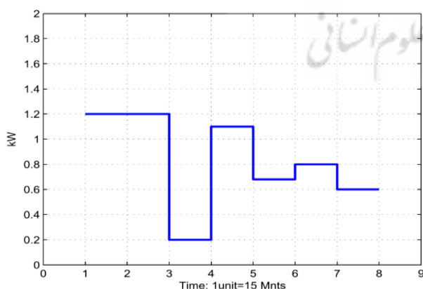
شکل ۱۰. پروفیل بار ماشین ظرف شویی
