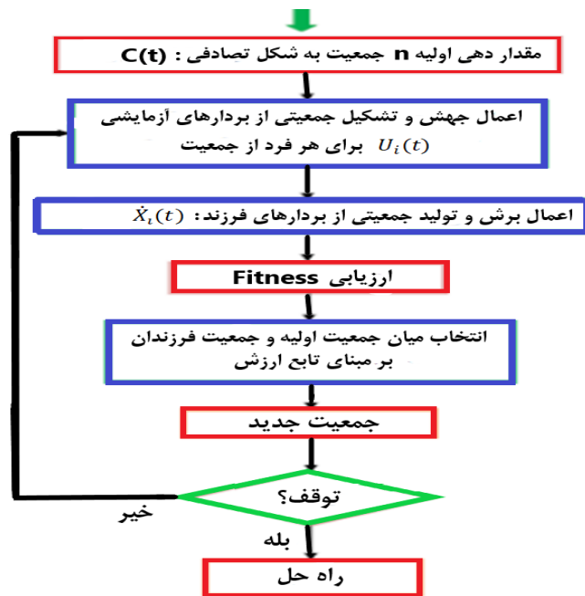
شکل ۵. فلوچارت الگوریتم DE
