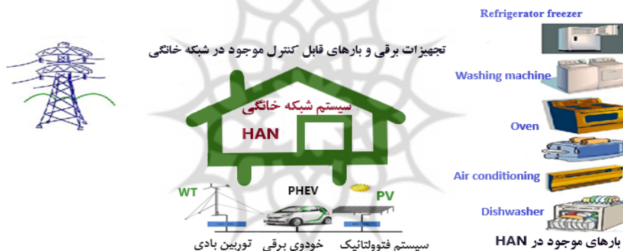
شکل ۶. سیستم شبکه خانگی در نظر گرفته شده
