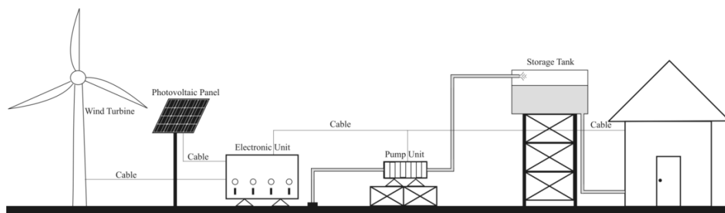
شکل ۵. طرحی شماتیک جهت بهره‌وری از انرژی‌های بادی و خورشیدی در شهر جیرنده
