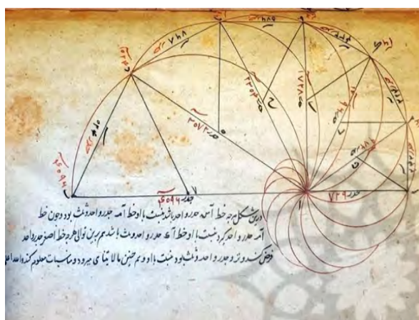
شکل ۵. روش ترسیم اعداد اصم به شیوه ی بوزجانی مأخذ: شهریار حاتمی، نهران بر عیان ، ۱۴۰۰
