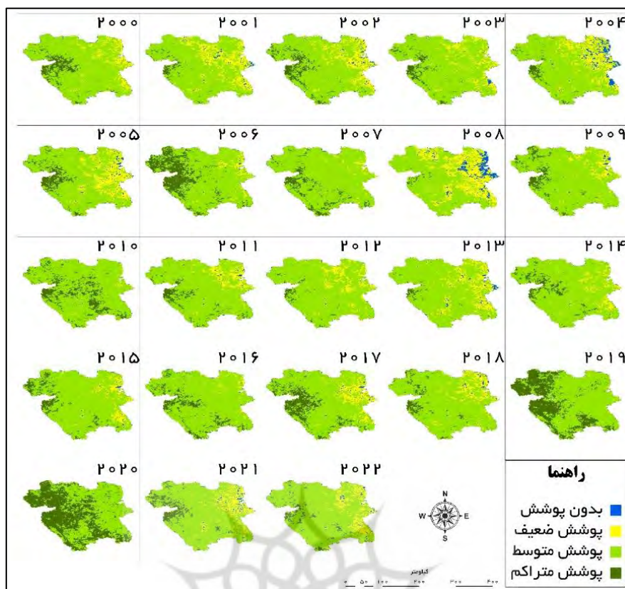
شکل ۲. طبقات پوشش گیاهی براساس شاخص NDVI در دوره آماری ۲۰۰۰ تا ۲۰۲۲
