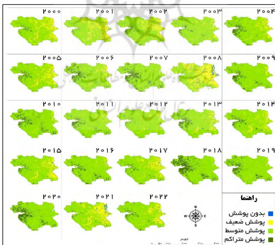
شکل ۳. طبقات پوشش گیاهی براساس شاخص EVI در دوره آماری ۲۰۰۰ تا ۲۰۲۲
