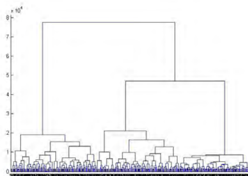
الف: دارنمای کلی
