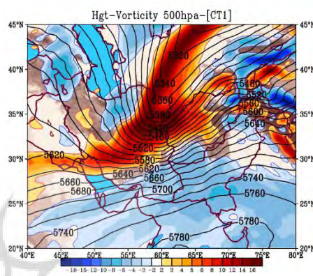
الف: وضعیت ارتفاع ژئوپتانسیل و تاوایی تراز ۵۰۰ هکتوپاسکال برای الگوی اول
