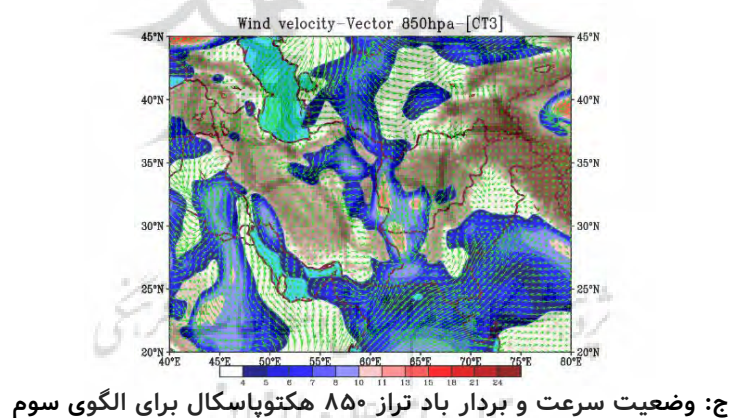
شکل ۷. وضعیت سرعت و بردار باد تراز ۸۵۰ هکتوپاسکال در دوره‌های گرد و غباری جنوب شرق ایران
