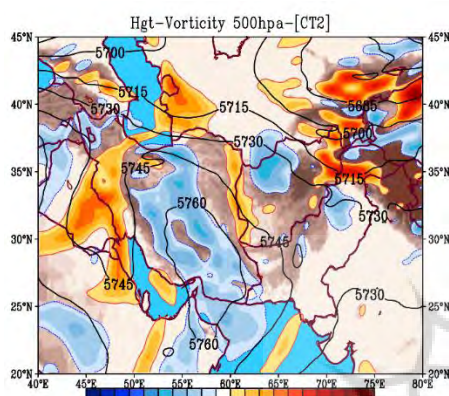
ب: وضعیت ارتفاع و تاوایی ژئوپتانسیل تراز ۵۰۰ هکتوپاسکال برای الگوی دوم
