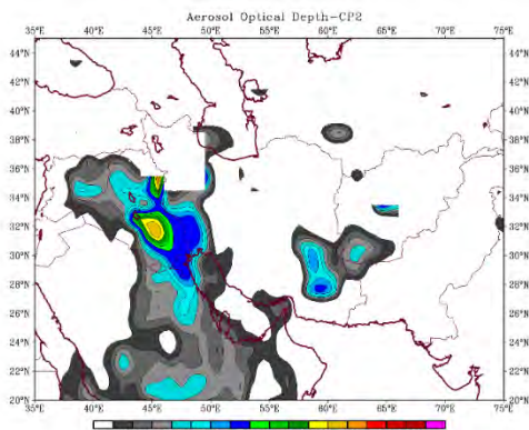
ب: وضعیت عمق اپتیکی آئروسول ۵۵۰ نانومتر الگوی دوم
