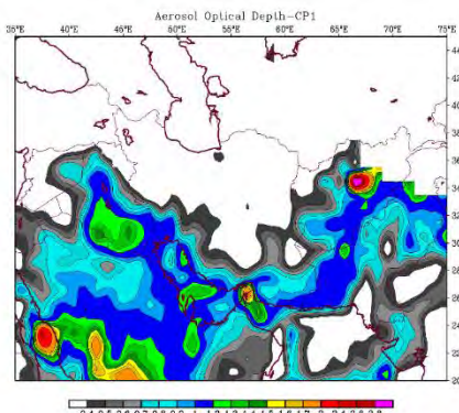
الف: وضعیت عمق اپتیکی آئروسول ۵۵۰ نانومتر برای الگوی اول
