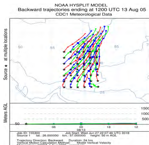
الف: ردیابی توده هوا برای الگوی اول-روز نماینده ۱۳ آگوست ۲۰۰۵
