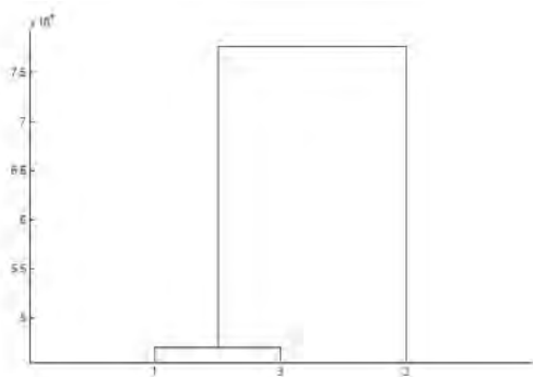
ب: دارنمای مربوط به ۳ الگوی گردشی
