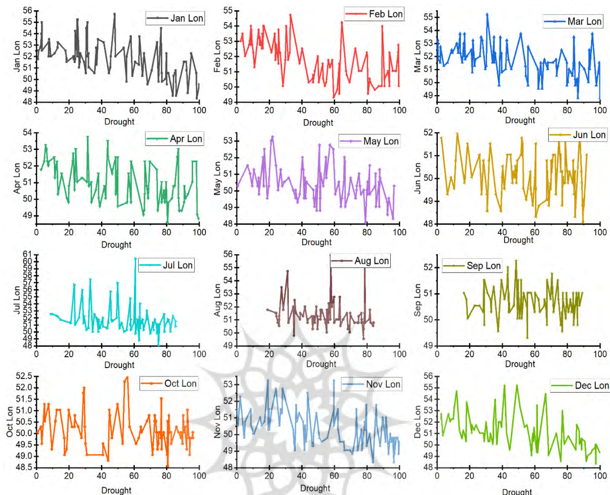
شکل ۶. ارتباط بین موقعیت طول جغرافیایی ثقل بارش ماهانه و درصد گستره خشکسالی ماهانه ایران (۱۹۴۰-۲۰۲۳)
