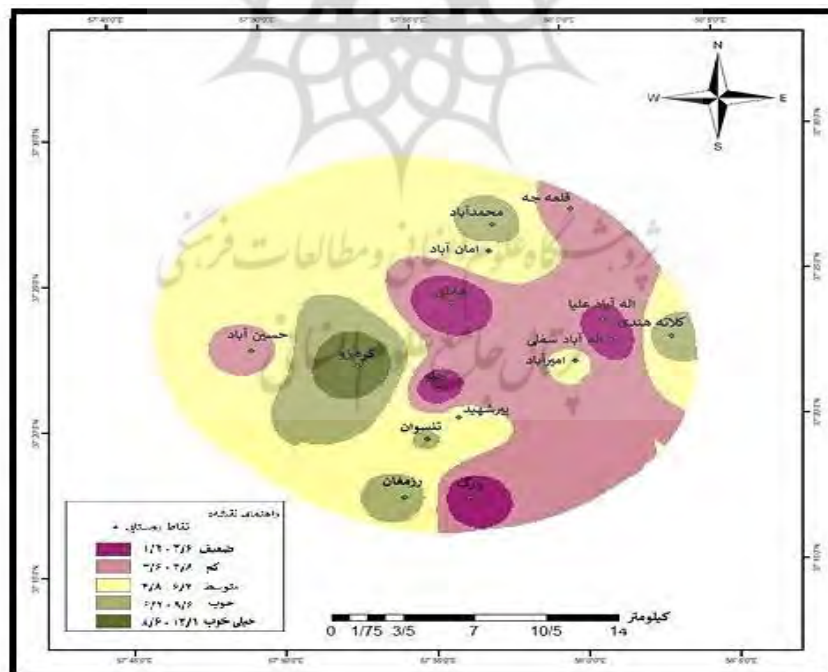
شکل ۲. تحلیل فضایی روستاهای مورد مطالعه از نظر وضعیت هویت مکانی در سکونتگاه‌های پیراشهری شیروان
