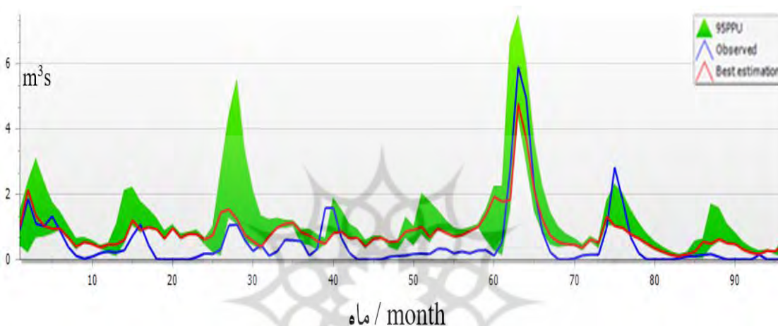
شکل ۶. هیدروگراف مشاهداتی و شبیه سازی شده رواناب ایستگاه دبی سنجی کرتیان در دوره اعتبارسنجی (۲۰۱۲-۲۰۲۰)
