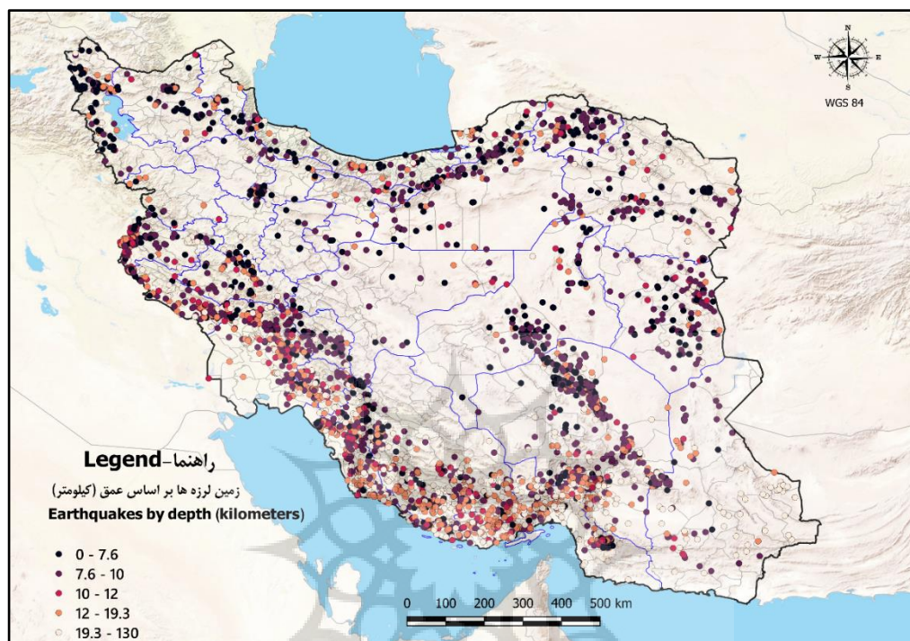
شکل ۴- پراکنش زمین‌لرزه‌های ایران بر اساس عمق (کیلومتر)
