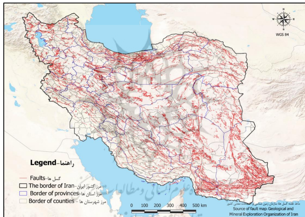
شکل ۱- پراکنش گسل های ایران Fig.1. Distribution of Faults in Iran
