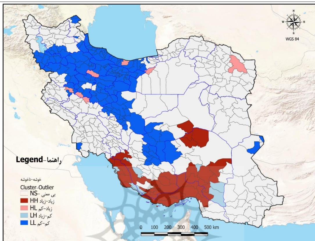
شکل ۷- نقشه خوشه-ناخوشه زمین‌لرزه‌های ایران (تحلیل موران محلی انسلین)
