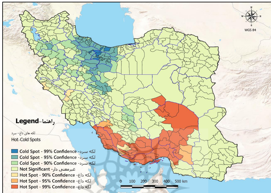
شکل ۶- نقشه لکه‌های داغ و سرد زمین‌لرزه‌های ایران Fig.6. Hot and Cold Spots Map of Earthquakes in Iran
