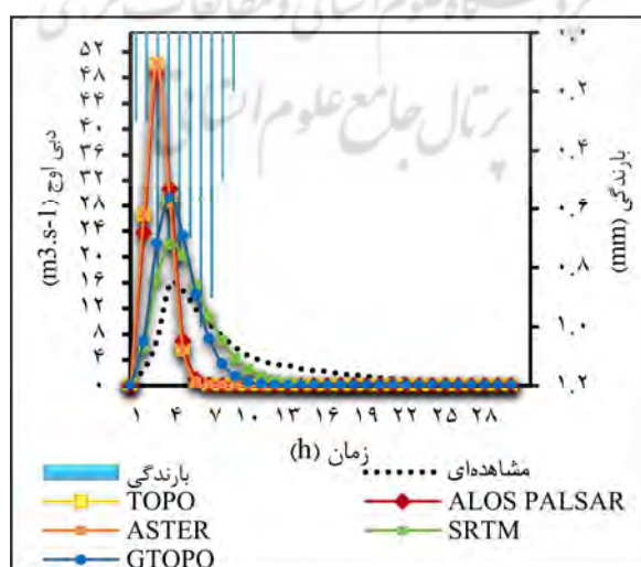
شکل ۶. نمونه‌ای از هیدروگراف تخمینی به‌روش رسو، در حوضه آبخیز کسلیان
