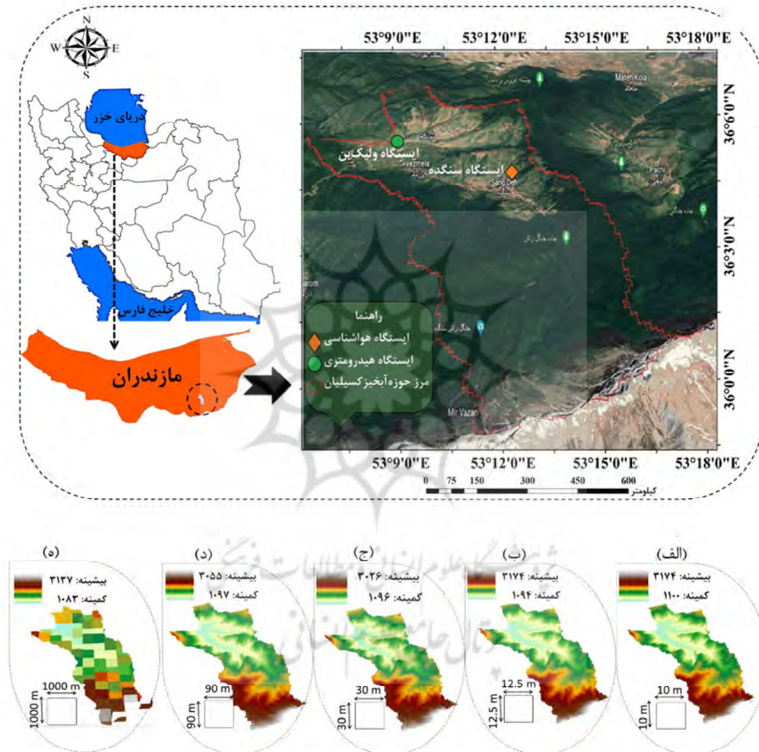
شکل ۱. موقعیت مکانی حوضه آبخیز کسلیان در ایران و مدل‌های رقومی ارتفاع متفاوت
