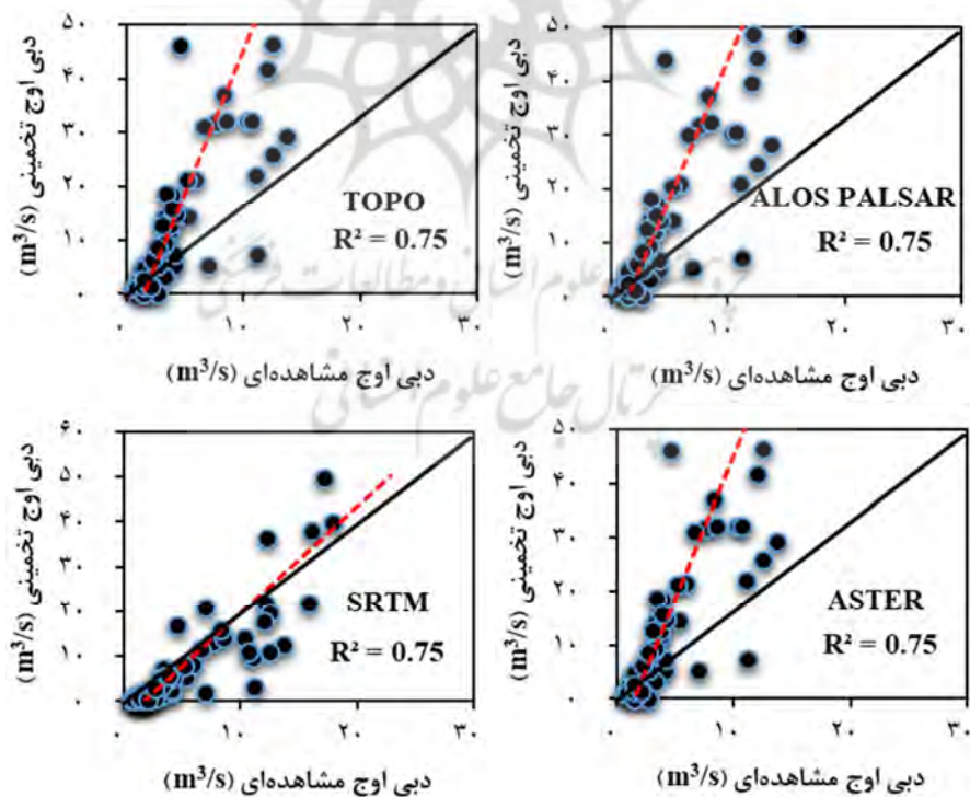
شکل ۴. مقایسه مقادیر برآوردی و مشاهده‌ای دبی اوج به‌روش روسو، با استفاده از مدل‌های متفاوت رقومی ارتفاع. خط مشکی بیانگر خط ۱:۱ و خط چین قرمز خط رگرسیون است
