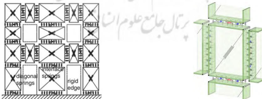
تصویر ۱ پ: درشت المان به کار گرفته شده در نرم افزار هیسترا (راست)، ساخت مدل دیوار بنایی با استفاده از درشت المان (چپ) (Chácara, 2018)
