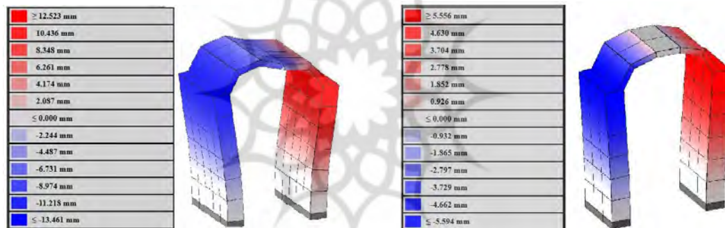
تصویر ۴: تغییرات جابجایی جانبی تحت بار ثقی در نمونه ایوان خانه‌های صفوی (راست) و آل مظفر (چپ)
