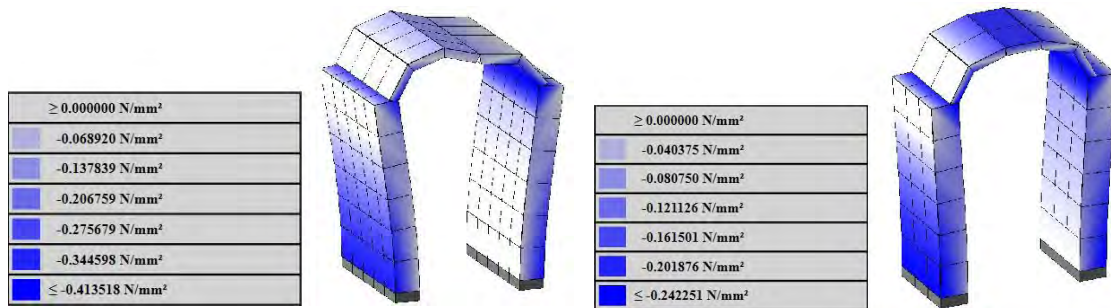
تصویر ۲: تغییرات تنش اصلی فشاری تحت بار ثقی در نمونه ایوان خانه‌های صفوی (راست) و آل مظفر (چپ)
