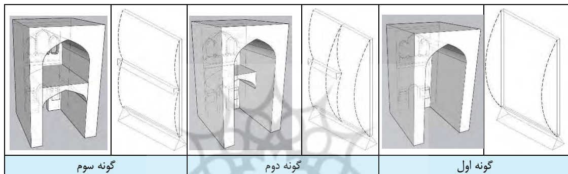
جدول ۸: گونه‌های مهار جانبی (عمود بر صفحه) جرز ایوان خانه‌های آل مظفر یزد (مأخذ: نگارندگان)
