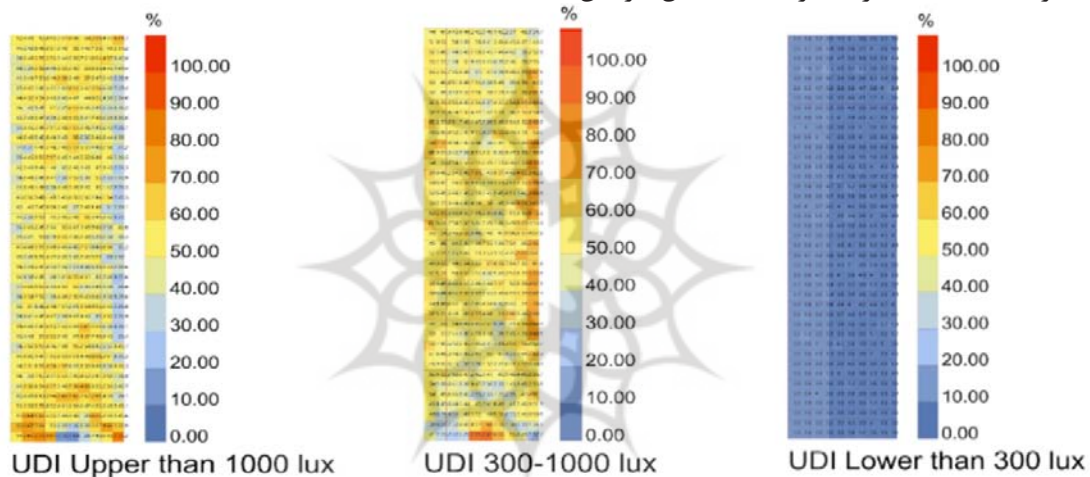
تصویر ۷. نمودارهای شاخص UDI در گلخانه با الگو دوم. مأخذ: نگارندگان.
