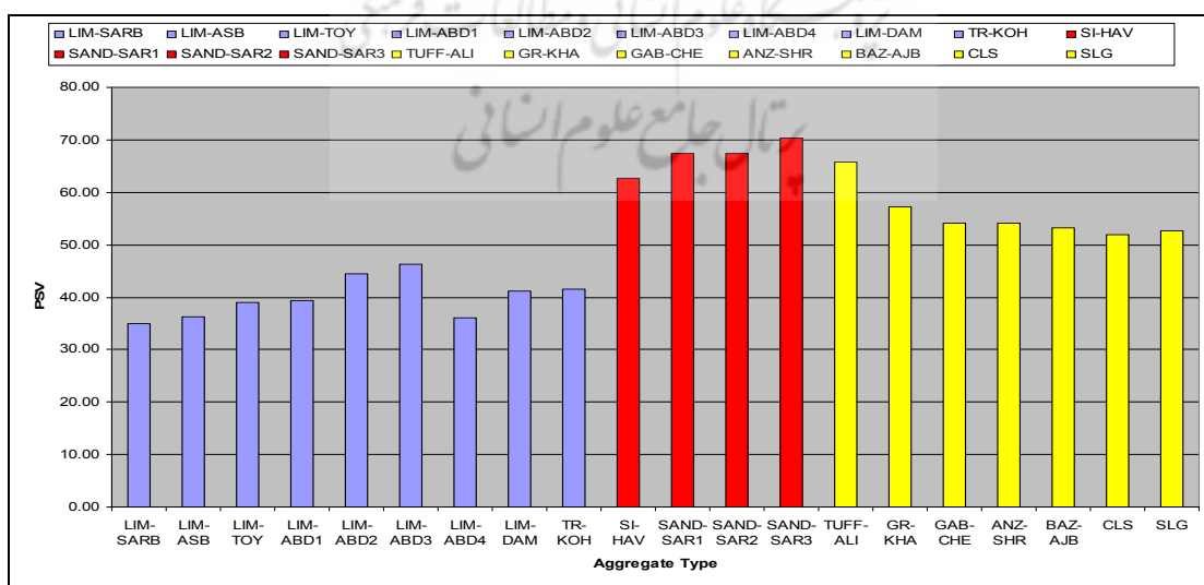
شکل ۷. مقادیر ارزش صیقلی سنگ (psv) برای سنگدانه های مختلف
